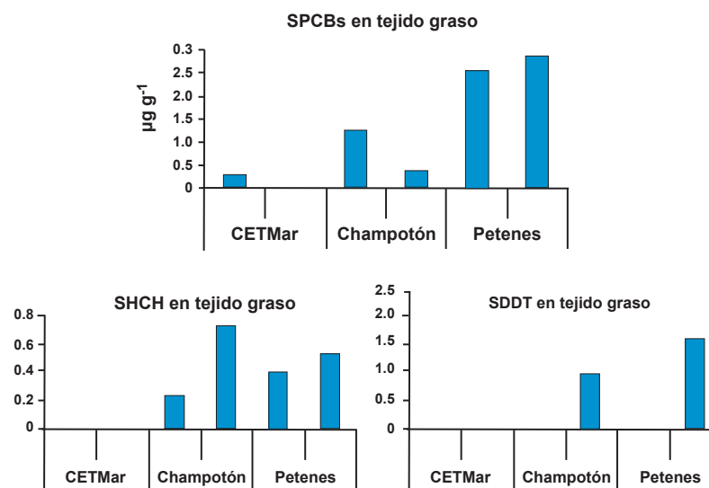
Figura 4. Residuos de \Sigma\text{PCBs} , \Sigma\text{HCHs} y \Sigma\text{DDT} en tejido graso de cocodrilo de río ( C. moreletti ) en Campeche.
